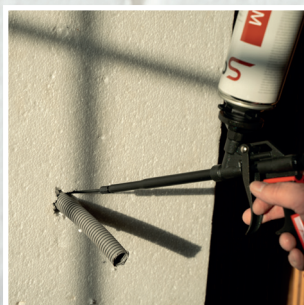
Durchbrüche ausspritzen
