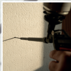
Dämmplatten fixieren
